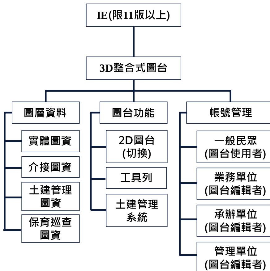
圖 3-2 玉山整合式圖台系統架構圖(IE 瀏覽器版本)
