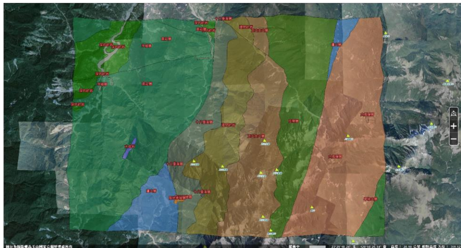
圖 3-14 區地地質圖
