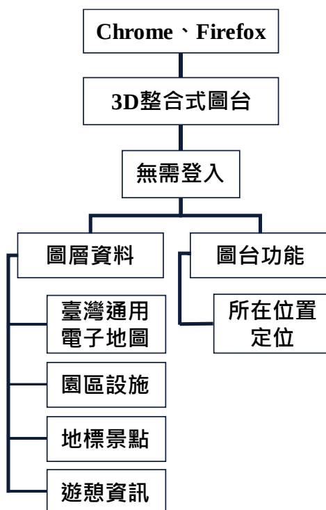
圖 3-67 圖台系統架構圖(跨瀏覽器版本)
