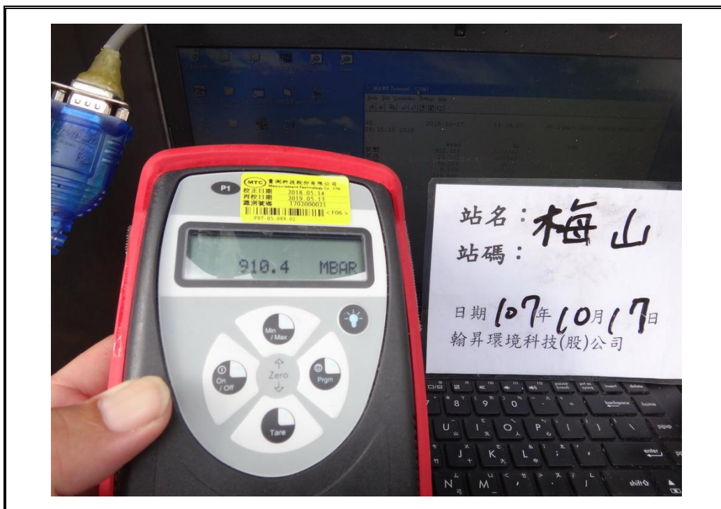
圖 11：梅山站氣壓比對
