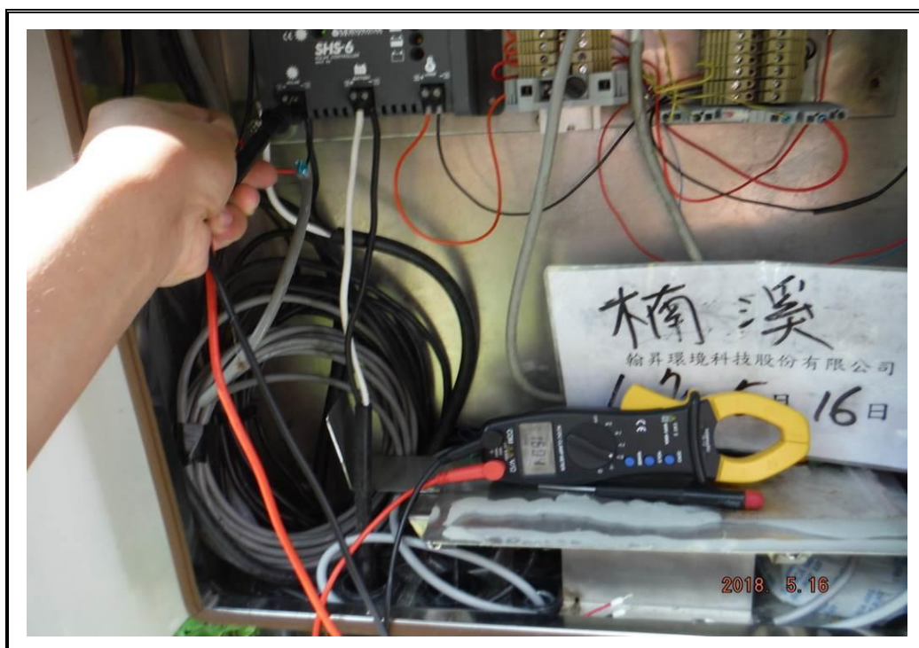
圖 2：楠梓仙溪站電源量測中
