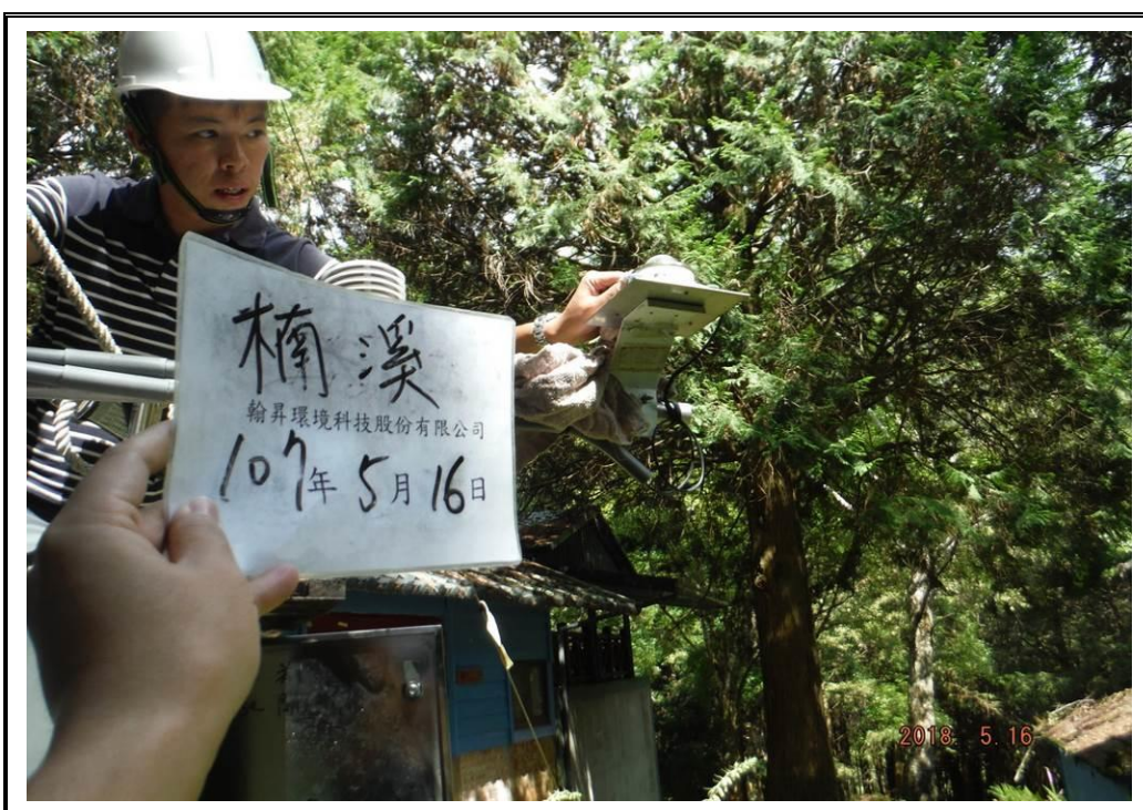
圖 6：楠梓仙溪站日照計清潔
