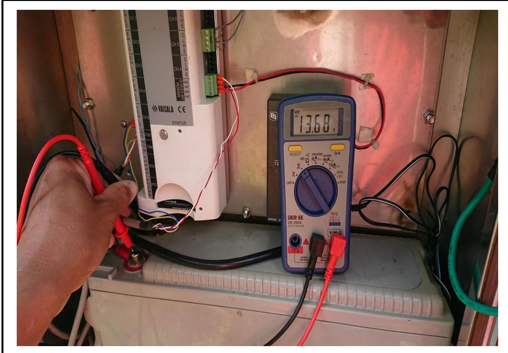
圖 11：大分站電壓量測
